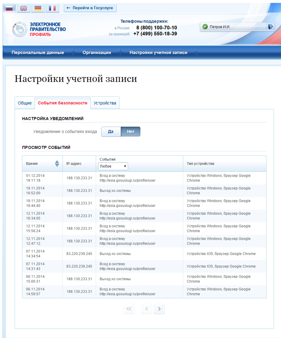
Рисунок 80 – События безопасности
