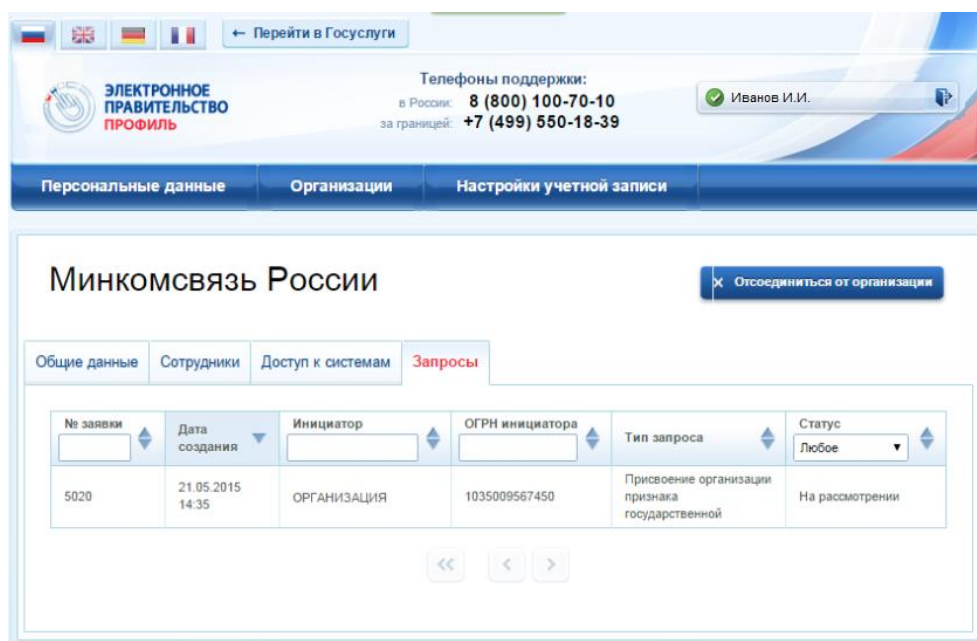
Рисунок 74 – Перечень заявок
